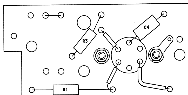
OSCILLATOR (BA 35195)
