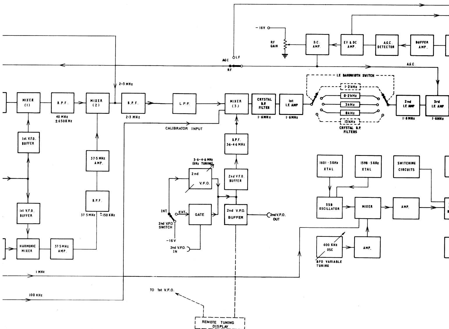
Block Diagram: R.A. 1217
