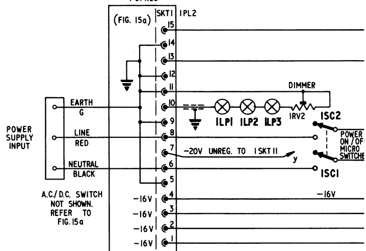
POWER SUPPLY MODULE PU. 1153
