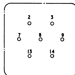
ITI TRANSFORMER TERMINALS
